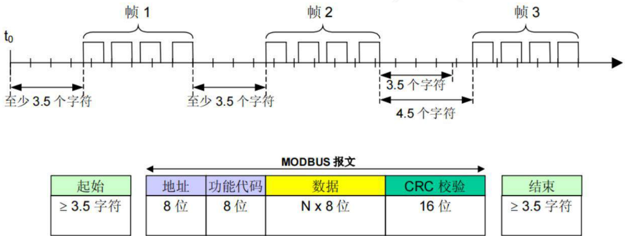
图 2-4 RTU 报文帧
