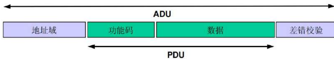
图 2-1 通用 MODBUS 帧
